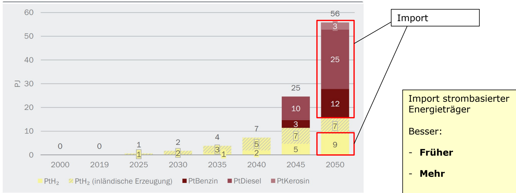
Abbildung 12: Verbrauch an strombasierten Energieträgern und inländische H 2 -Produktion
