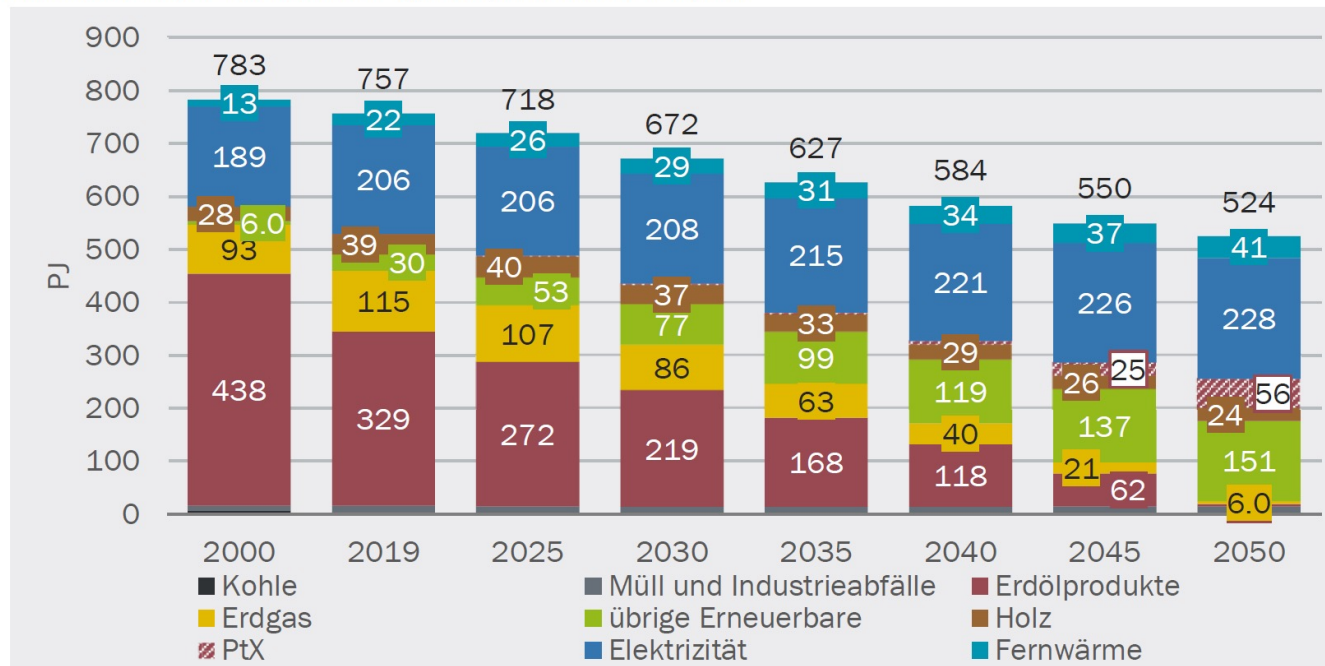
Abbildung 2: Entwicklung des Endenergieverbrauchs nach Energieträgern
